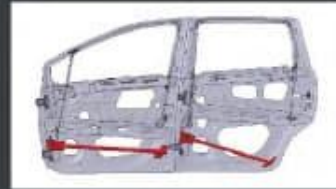
SIDE DOOR IMPACT BEAM คาบเหล็กนิรภัยกันกระแทกบริเวณแผงประตู เพื่อลดแรงปะทะจากด้านข้างให้กับผู้โดยสารในกรณีเกิดอุบัติเหตุ
